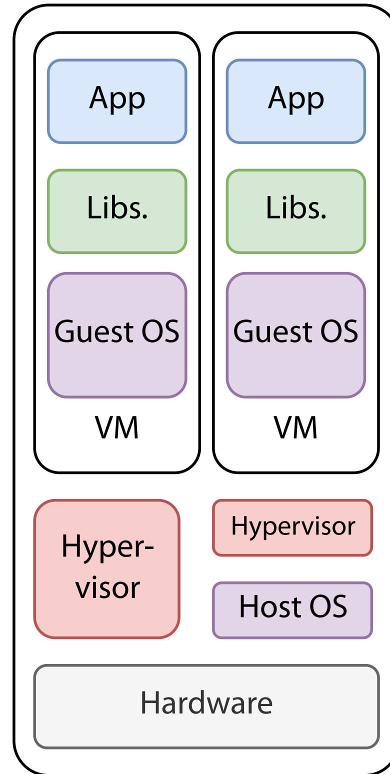
Virtuelle Maschine
