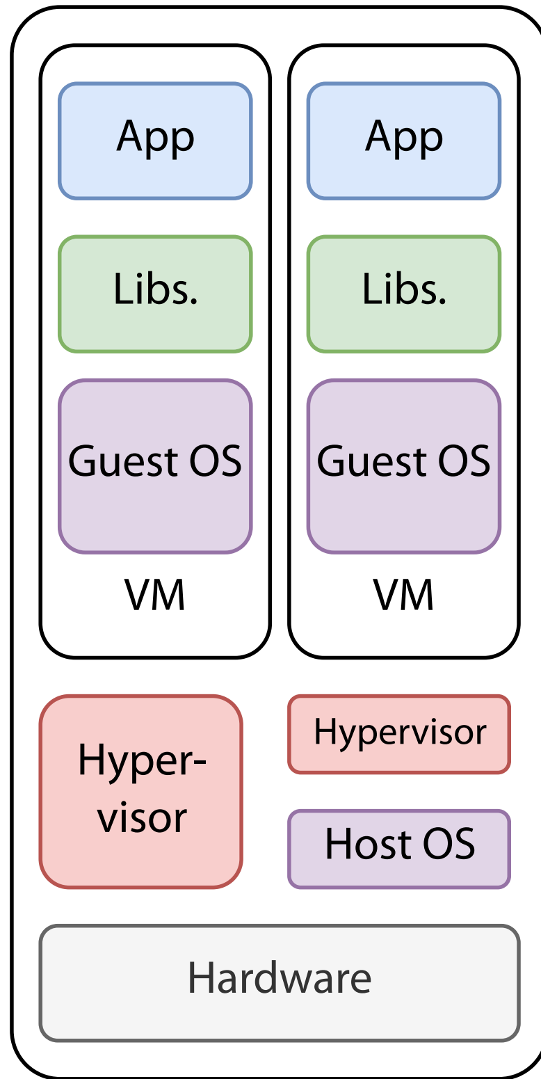
Virtuelle Maschine
